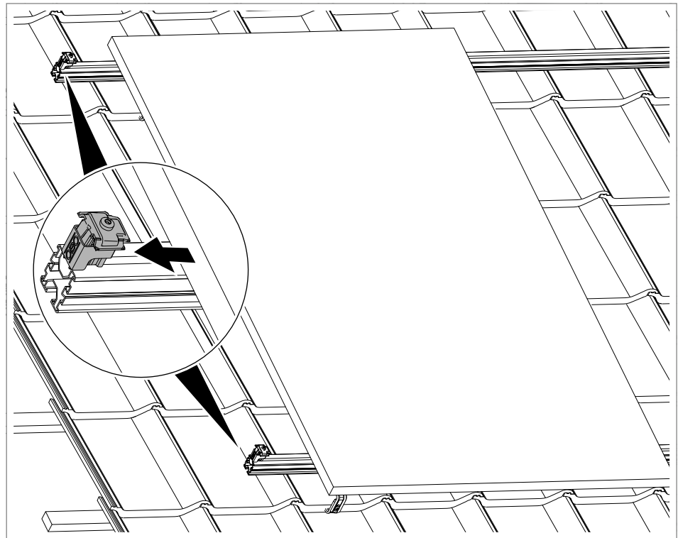
Abb. 17: PV-Modul auflegen
