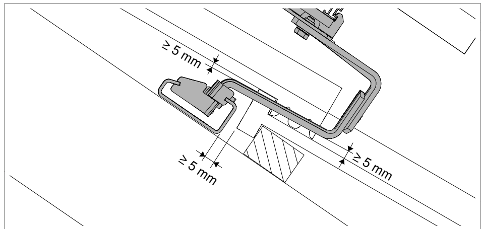
Abb. 7: Mindestabstände Dachhaken zu Ziegeln
