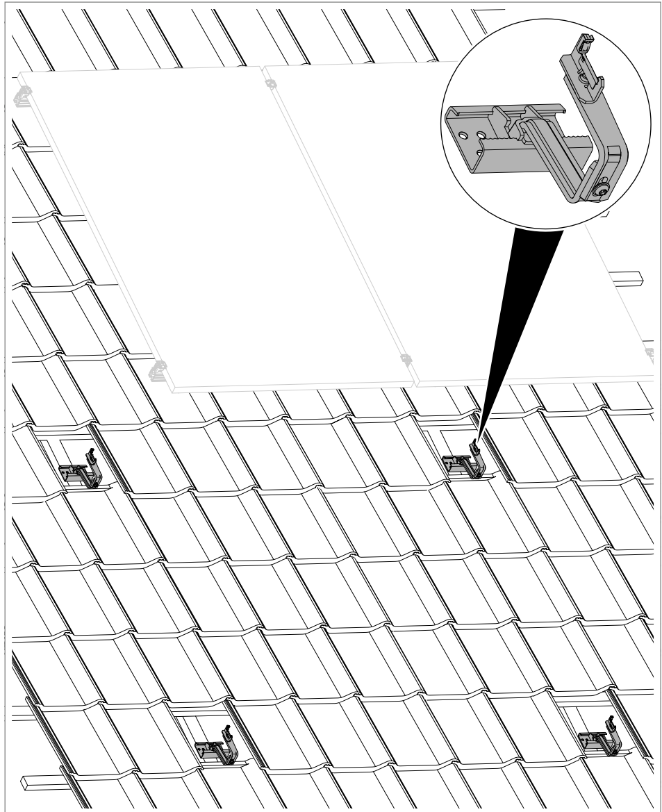
Abb. 4: Dachhaken positionieren
