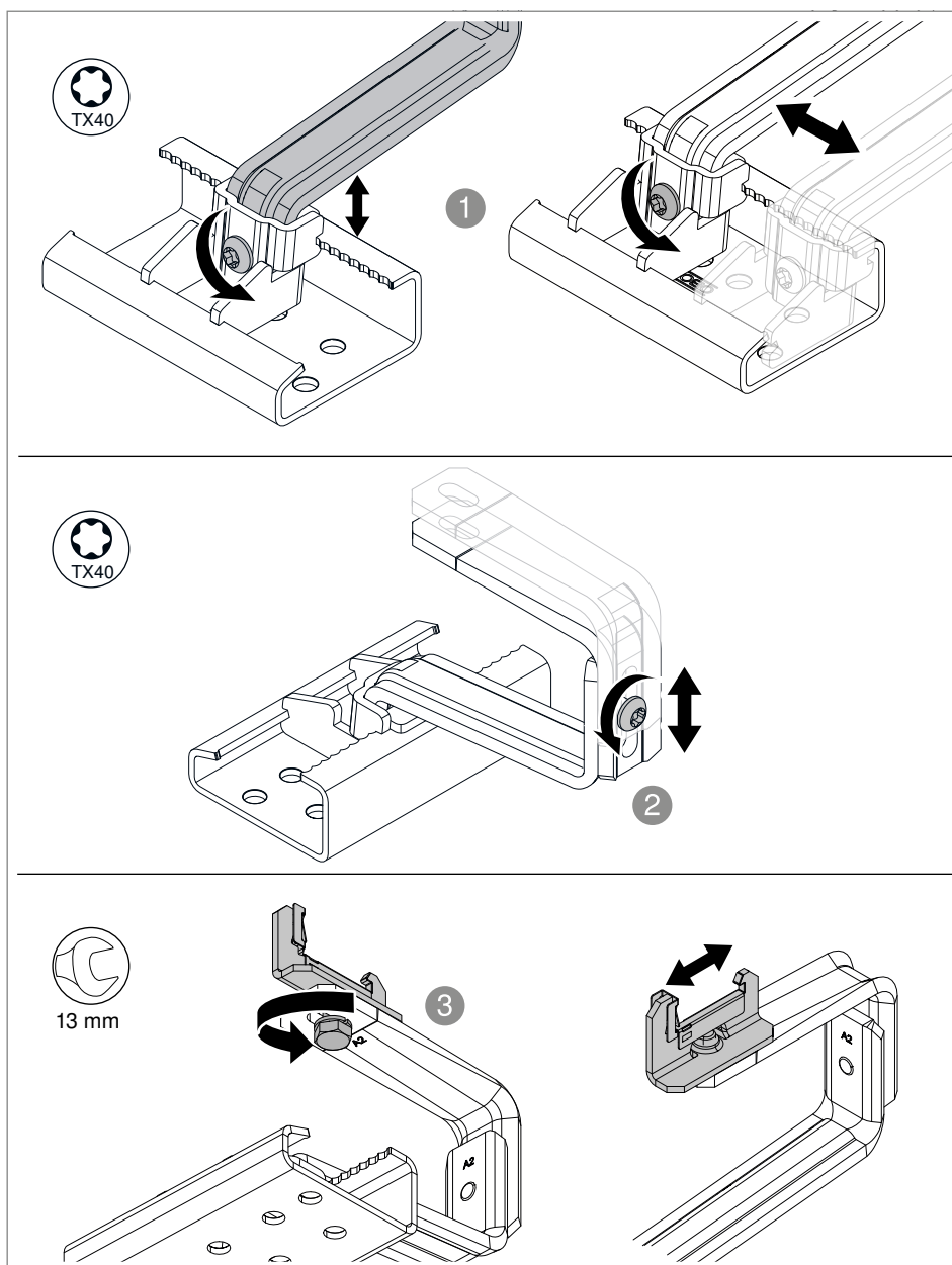
Abb. 6: Dachhaken einstellen
