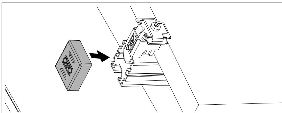
Abb. 25: Schutzkappe montieren
