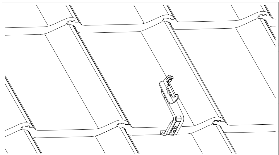
Abb. 14: Ziegel aufdecken
