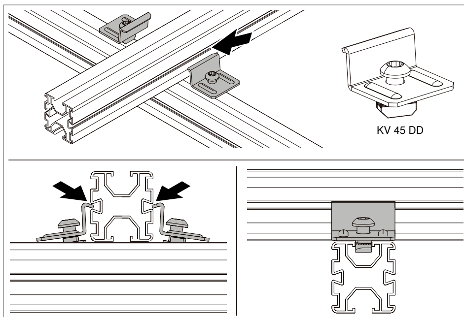
Abb. 30: Kreuzverbinder einsetzen
