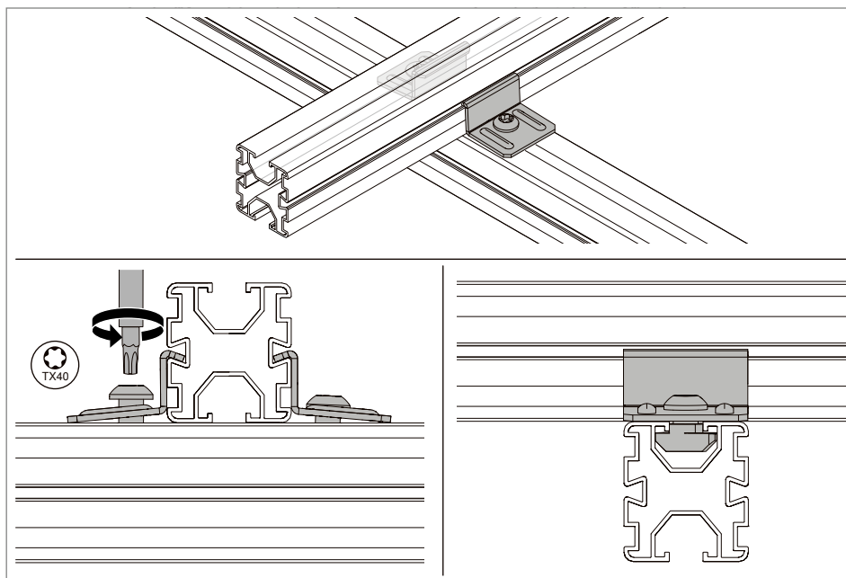
Abb. 31: Kreuzverbinder anschrauben
