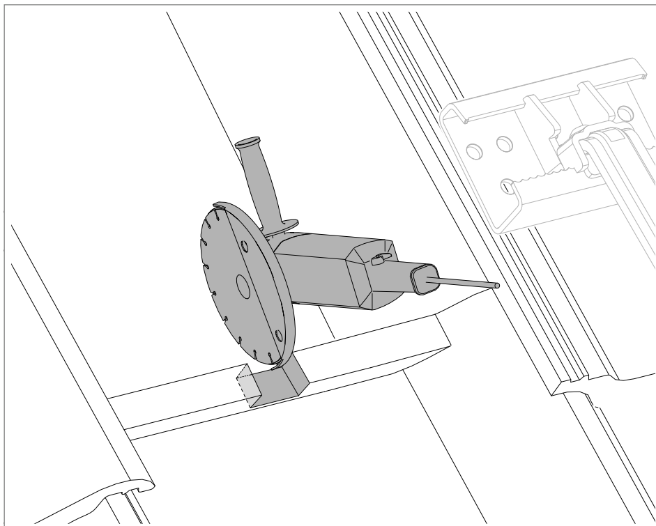
Abb. 9: Ziegel aussparen
