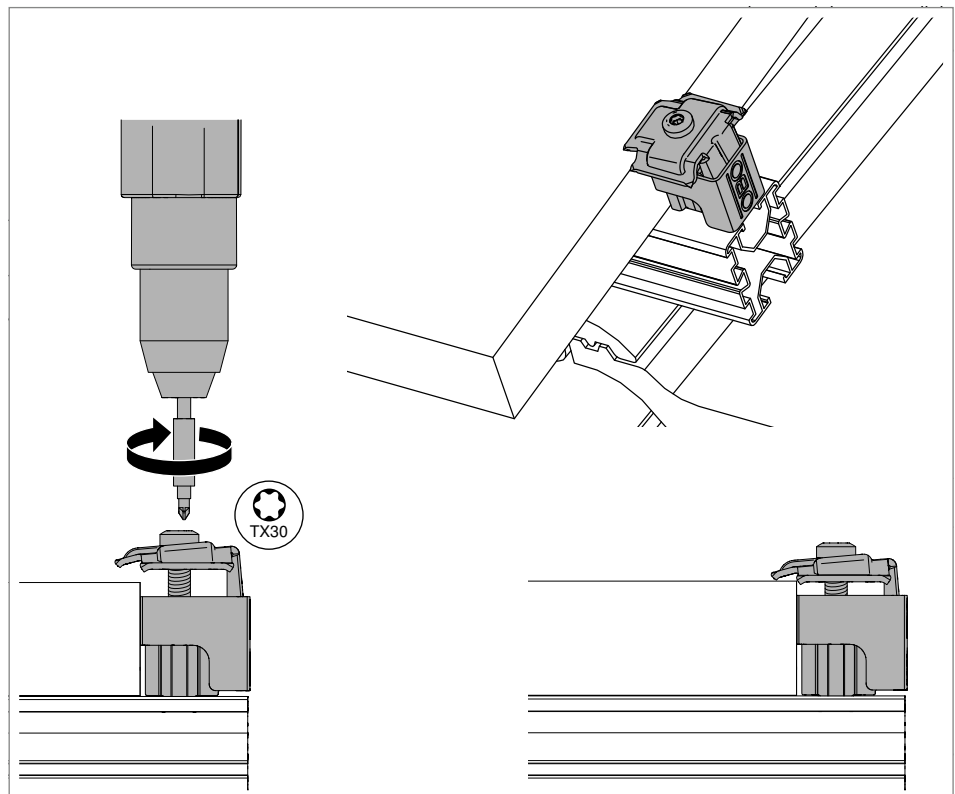
Abb. 22: Universalklemmen als Endklemme rechts anschrauben
