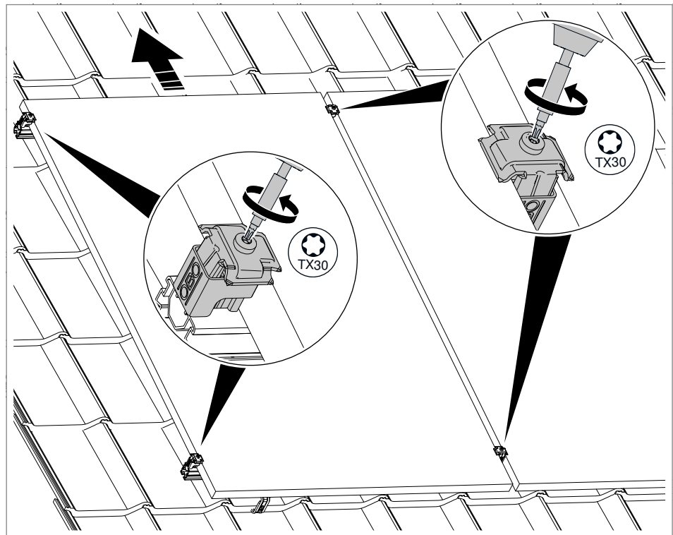
Abb. 23: Universalklemmen lösen
